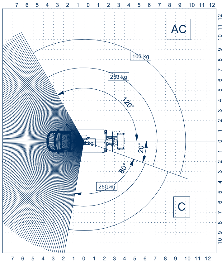
Einseitig abgestützt
